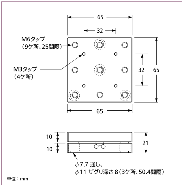
07 BKS 704 キネマチックベース
